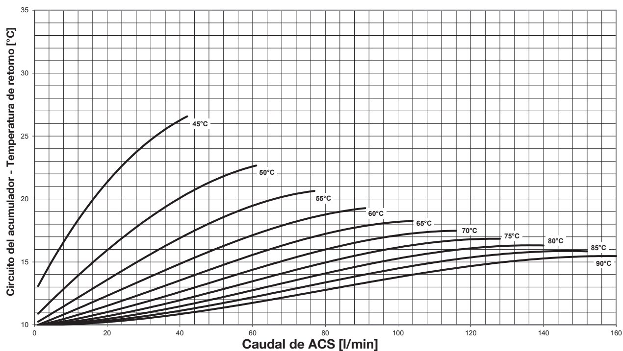
Temperatura de retorno del circuito del acumulador a diferentes temperaturas de caudal - Calentamiento de agua potable de 10°C a 45°C -
