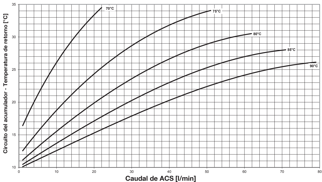
Temperatura de retorno del circuito del acumulador a diferentes temperaturas de caudal - Calentamiento de agua potable de 10°C a 70°C -
