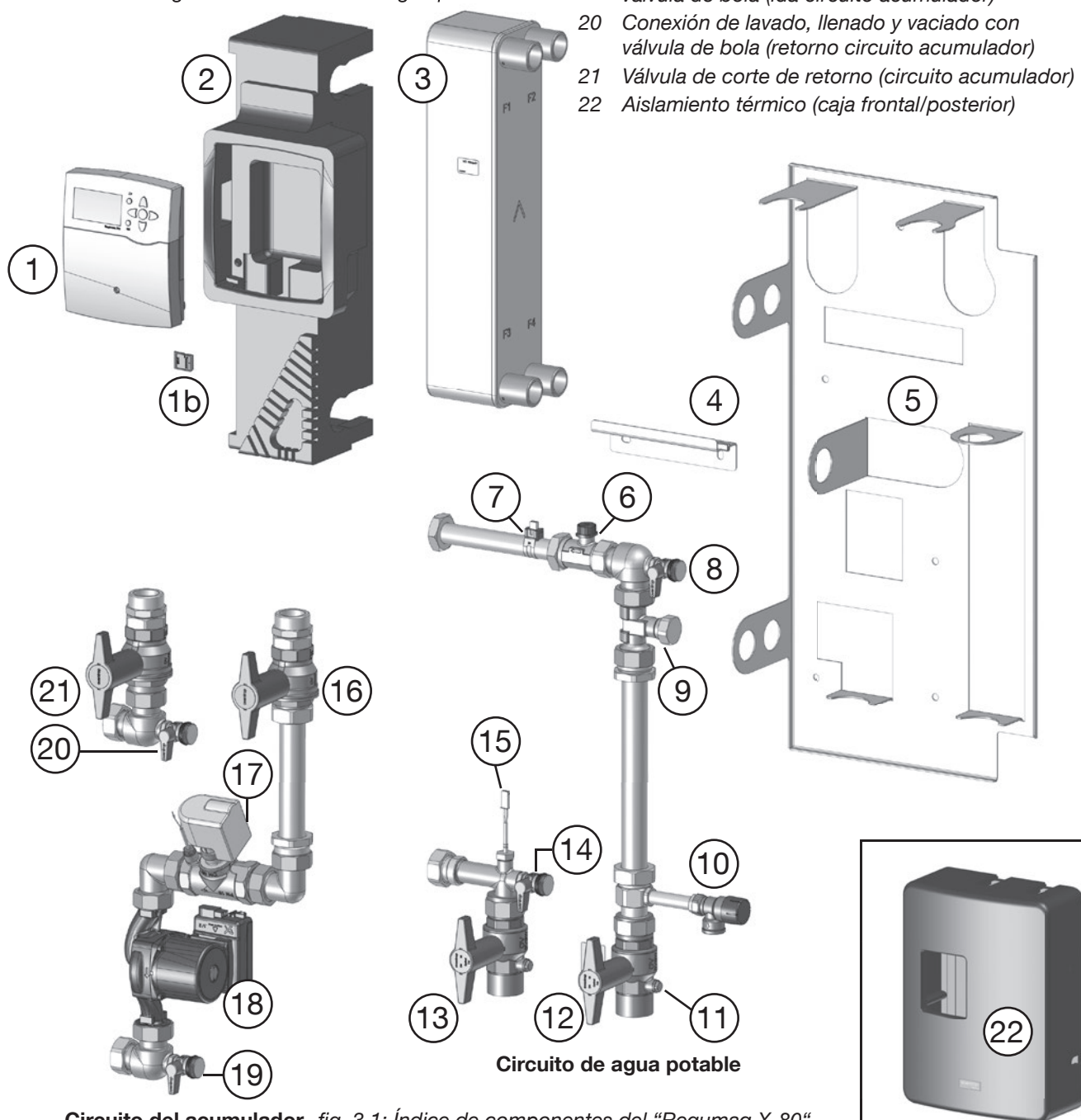
Circuito del acumulador fig. 3.1: Índice de componentes del “Regumaq X-80”
