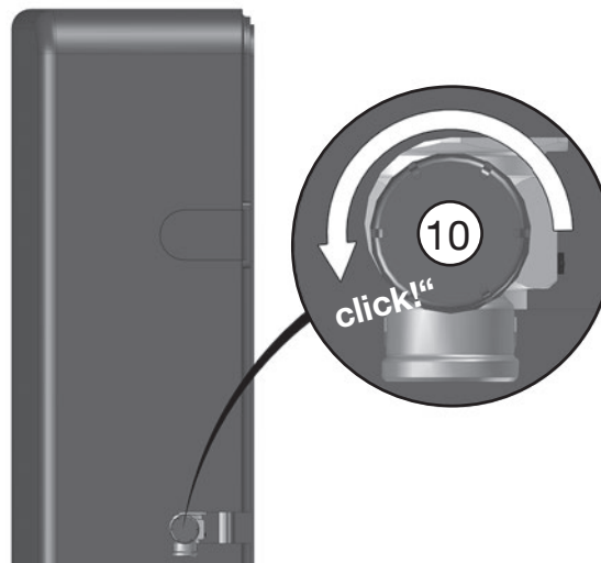
fig. 6.4: Gire la válvula de seguridad en sentido antihorario
