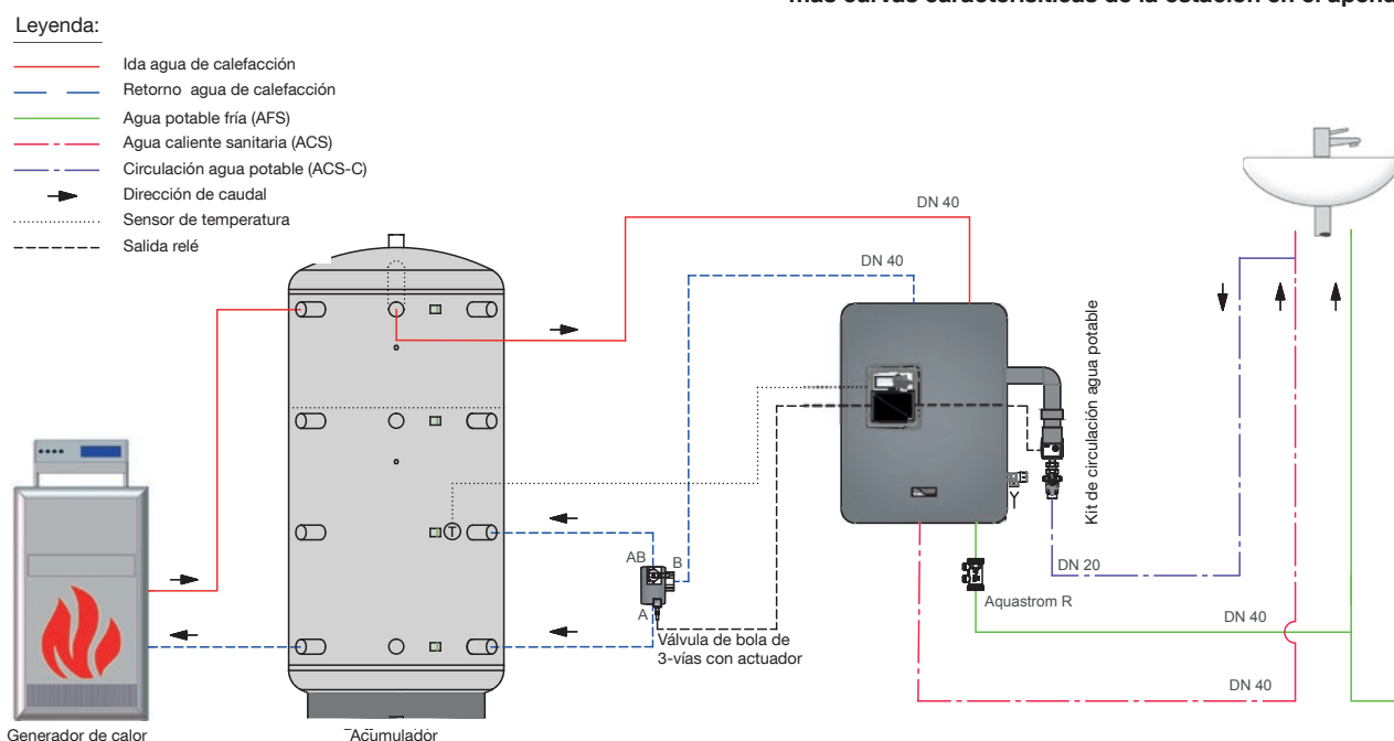
fig. 3.5: Diagrama de sistema con una estación de agua potable “Regumaq X-80”
