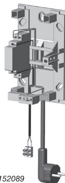
fig. 3.10: Kit de circulación de agua potable, art. n° 1381590
