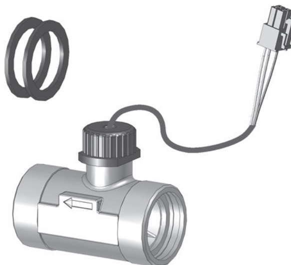
fig. 3.24: Sensor de caudal (repuesto circuito de agua potable), VTH 25; art. n° 1381593
