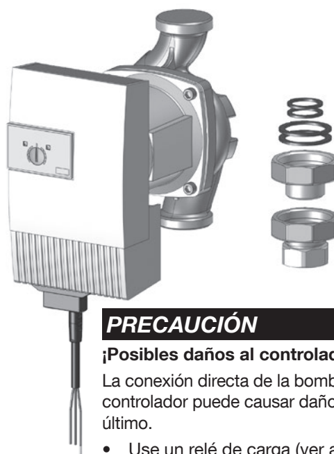
fig. 3.12: Bomba de circulación Wilo Stratos (12 m), art. n° 1381592
