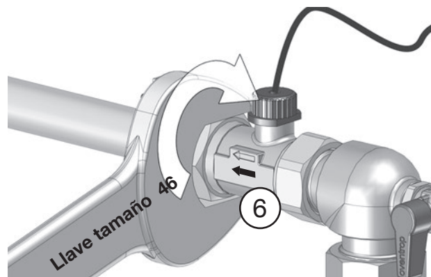
fig. 5.16: Afloje las tuercas del sensor de caudal
