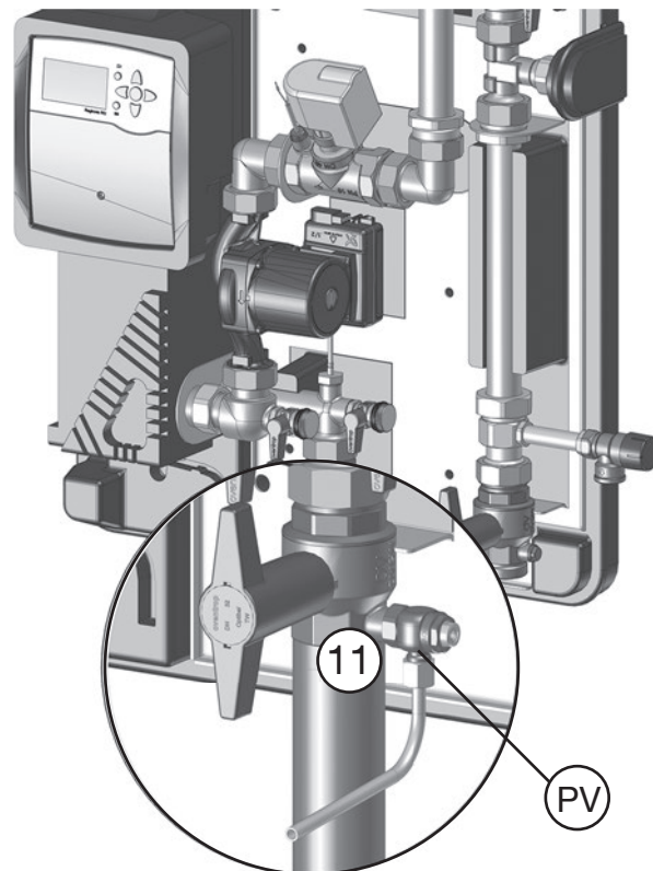
fig. 7.1: Conexión de la válvula toma de muestras a la estación
