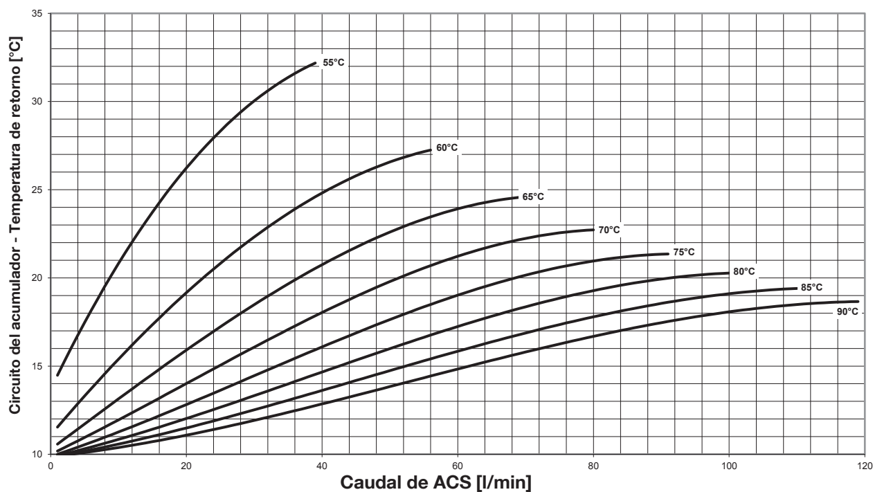
Temperatura de retorno del circuito del acumulador a diferentes temperaturas de caudal - Calentamiento de agua potable de 10°C a 55°C -
