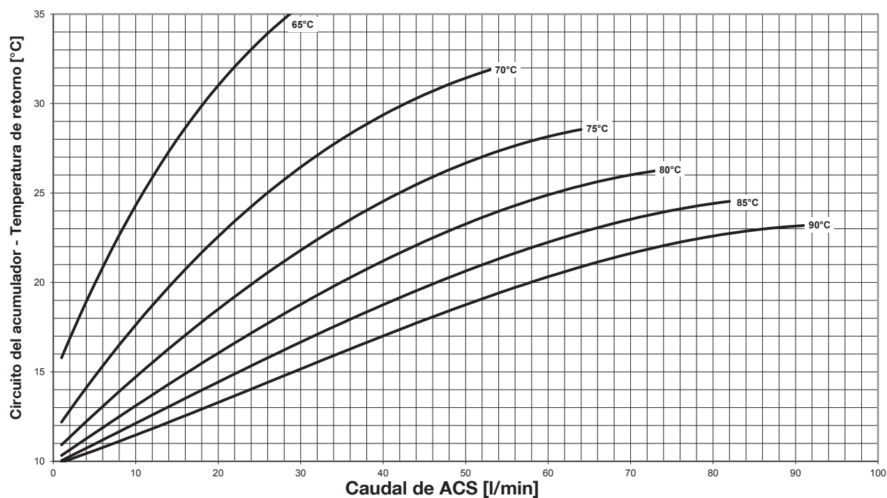
Temperatura de retorno del circuito del acumulador a diferentes temperaturas de caudal - Calentamiento de agua potable de 10°C a 65°C -
