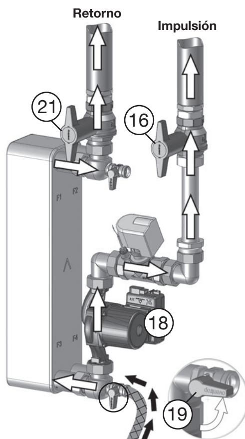
fig. 4.15: Llenado y purgado del circuito del acumulador
