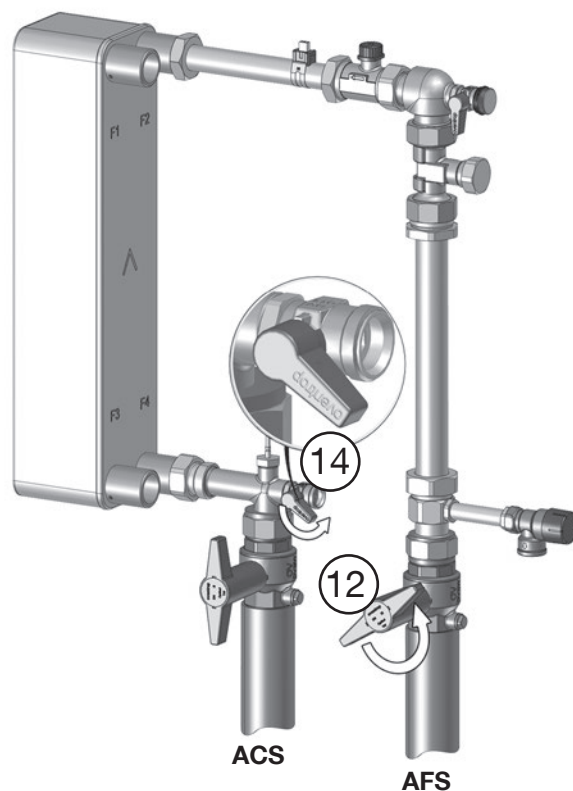
fig. 4.17: Llenado del agua fría (AFS)
