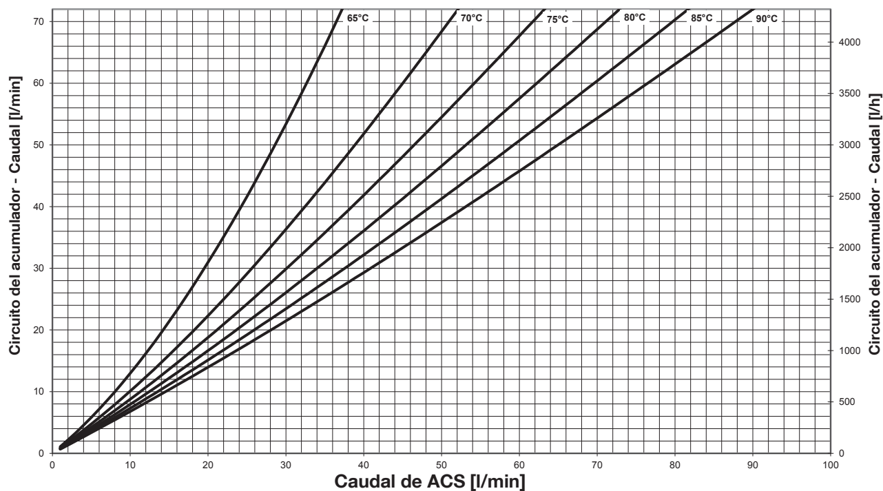
Caudal del circuito del acumulador a diferentes temperaturas de caudal - Calentamiento de agua potable de 10°C a 65°C -
