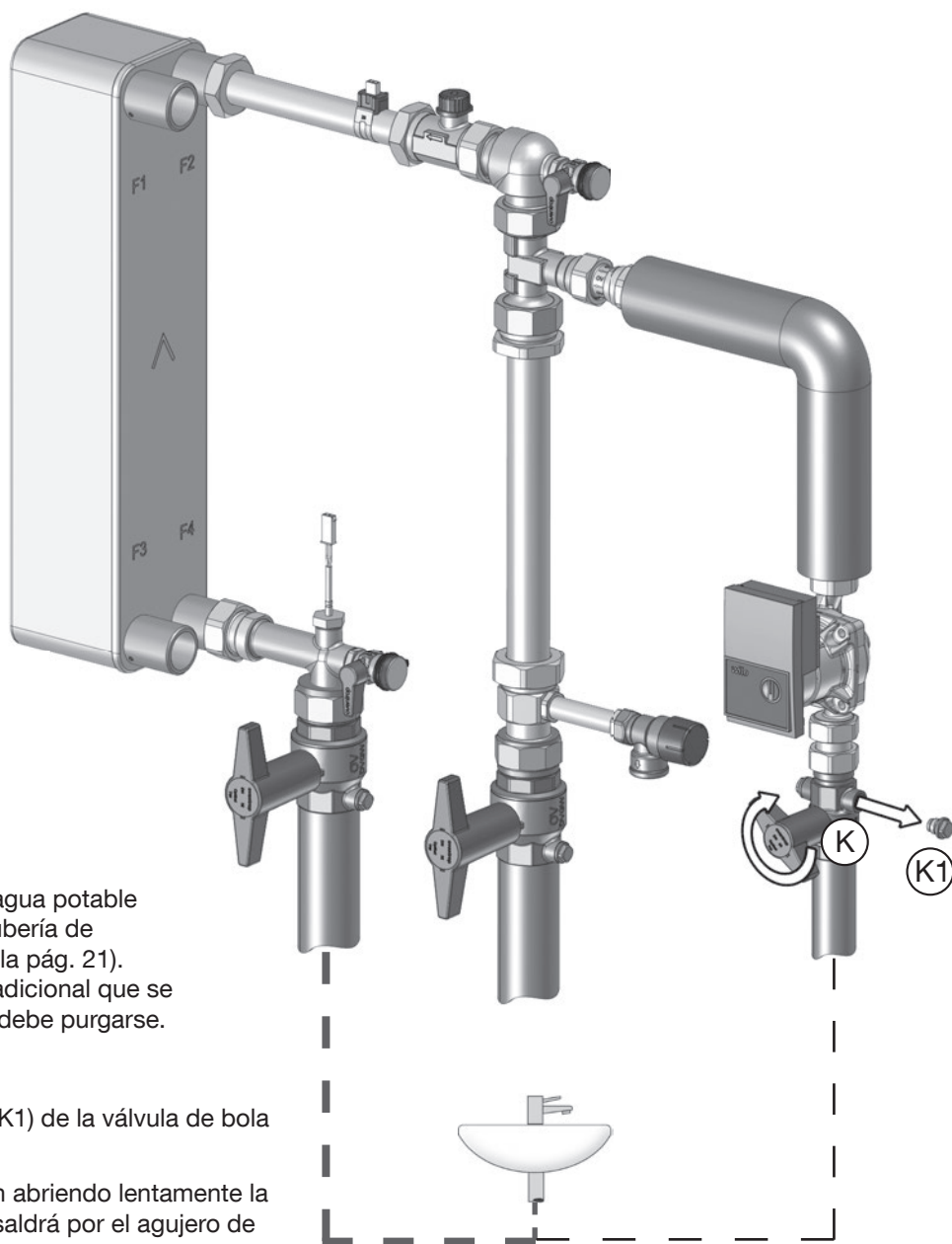
fig. 4.18: Purgado de una tubería adicional de circulación
