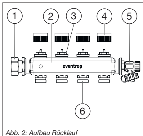
Abb. 2: Aufbau Rücklauf
