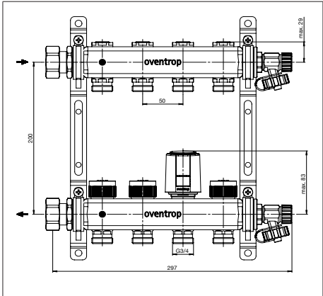
Abb. 5: Maße
