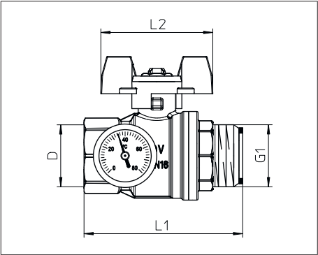
Abb. 6: Maße Kugelhahn
