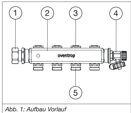
Abb. 1: Aufbau Vorlauf
