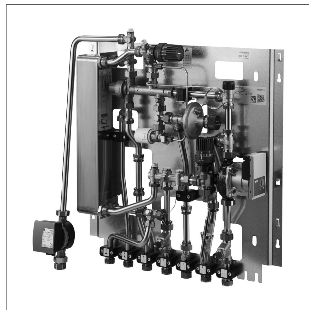
„Regudis W-HTF“-gemischter Heizkreis mit Zirkulationsleitung
