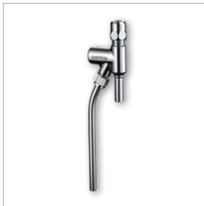
Aquastrom P monsterafnamekraan voor montage op hoekstopkraan
