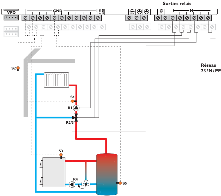
Schéma 8: circuit de chauffage mélangé avec chaudière à combustible solide
