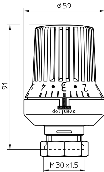
Abb. 2: Abmessungen Thermostat
