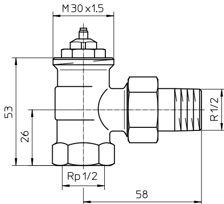
Abb. 1: Abmessungen Thermostatventil
