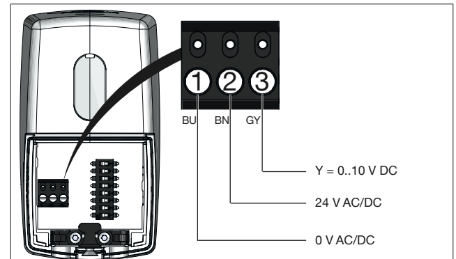
Abb. 6: Anschlussbelegung stetige Ansteuerung
