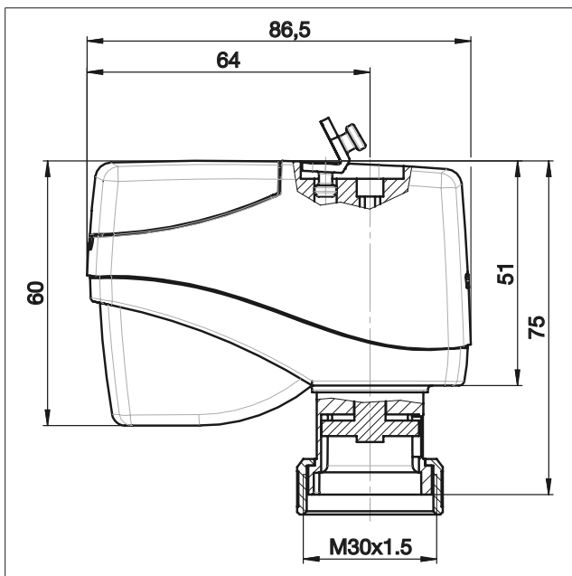
Abb. 2: Seitenansicht
