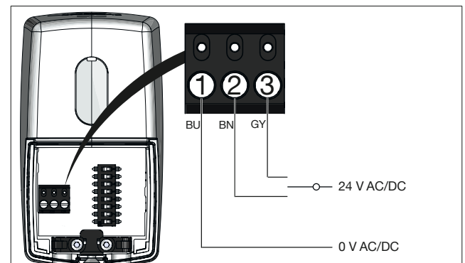
Abb. 7: Anschlussbelegung 3-Punkt Ansteuerung
