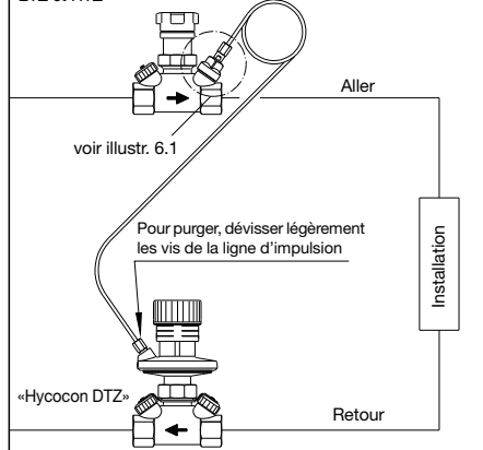
Illustr. 6.2: «Hycoco DTZ» Montage sur le retour
