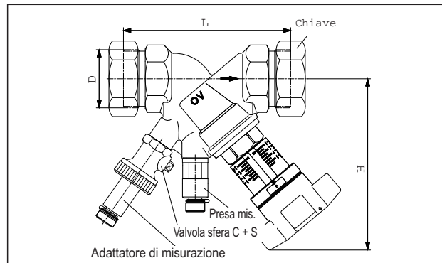
Dimensioni „Hydrocontrol VPR“
