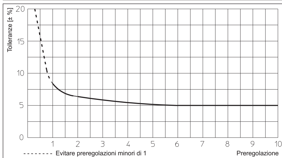
Tolleranze di portata dipendenti dalla preregolazione per 106 01/02/03/05, DN 10 fino a DN 50
