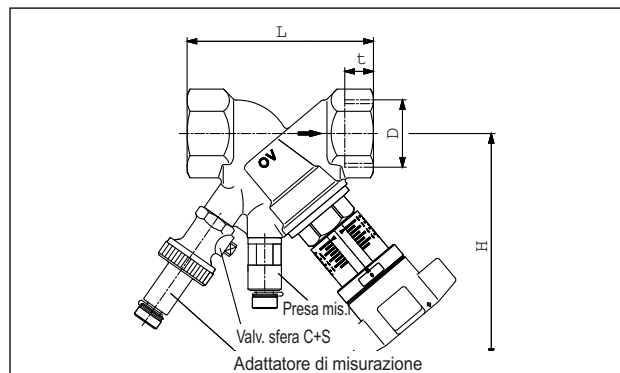
attacchi filettati femmina sec. EN, cod. art.: 106 01 . .
