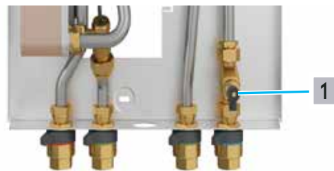
Abb. 28: Position Filtereinsatz Heizkreis-Rücklauf
