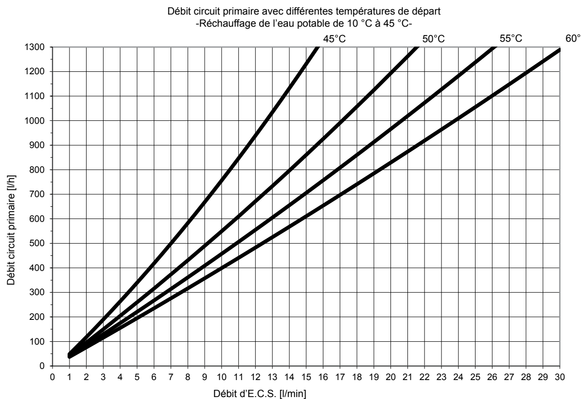
Fig. 40: Plage de puissance 2, réchauffage de l'eau potable à 45 °C
