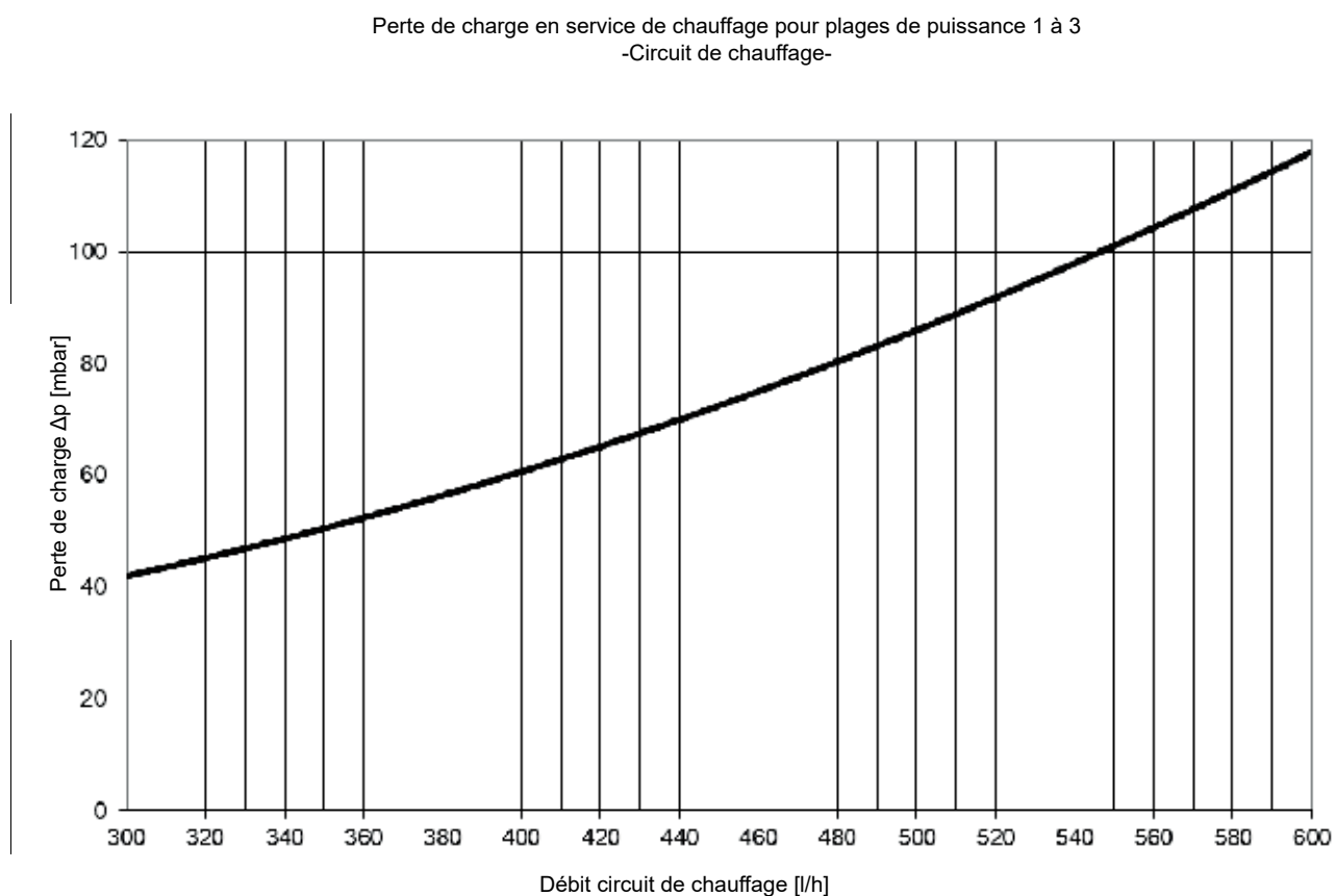
Fig. 32: Perte de charge dans le circuit primaire
