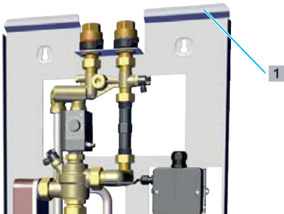
Fig. 19: Montage du capot pour pose en applique
