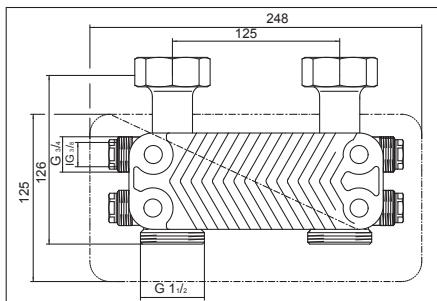
Теплообменник „Regumat“
