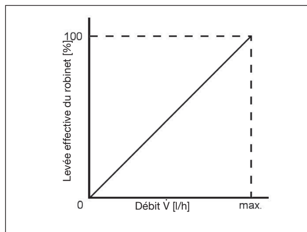
Courbe de fonctionnement du robinet «Cocon QTR»
