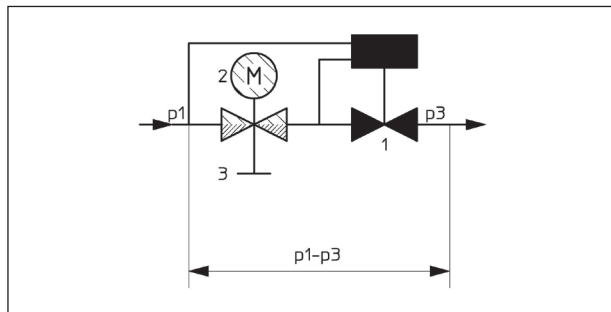
Pression différentielle
