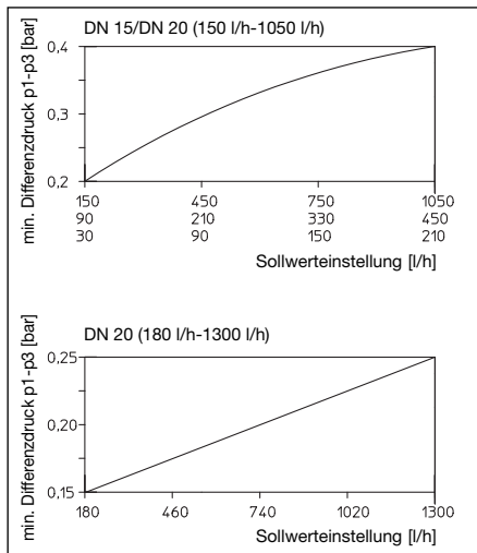
Abb. 5.7 Min. Differenzdruck / Sollwertereinstellung
