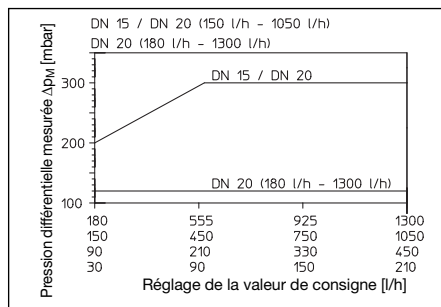
Fig. 5.1 Pression différentielle / Réglage de la valeur de consigne
