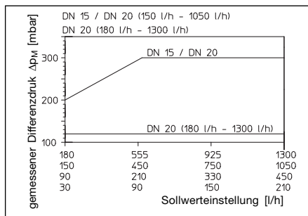
Abb. 5.1 Differenzdruck / SollwertEinstellung
