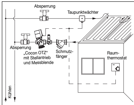
Abb. 6.1 Zweileitersystem
