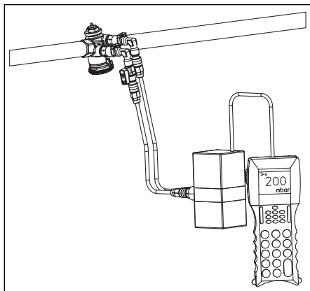
Abb. 5.5 Differenzdruckmessung
