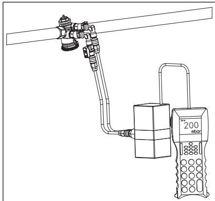
Fig. 5.5 Mesure de la pression différentielle
