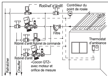
6.2 Système à quatre tuyaux
