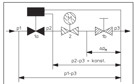
Abb. 5.3 Funktionsprinzip „Cocon QTZ“
