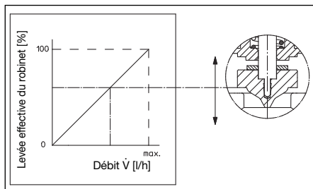
Fig. 5.4 Courbe de fonctionnement de l'unité de régulation de «Cocon Q»
