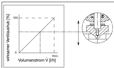
Abb. 5.4 Kennlinie der Reguliereinheit des „Cocon Q“
