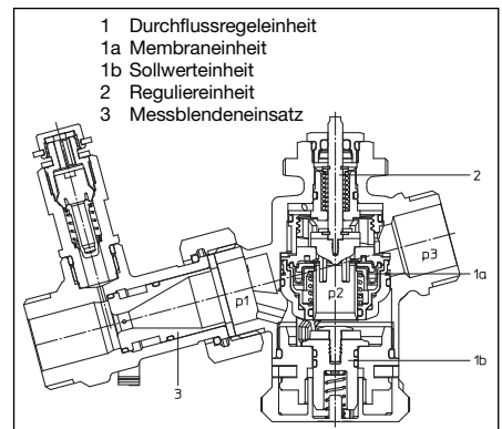
Abb. 5.2 Aufbau „Cocon QTZ“ mit Messblende
