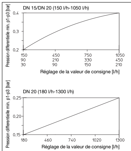
Fig. 5.7 Pression différentielle min. / Réglage de la valeur de consigne
