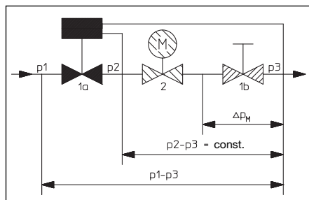
Fig. 5.3 Principe de fonctionnement «Cocon QTZ»
