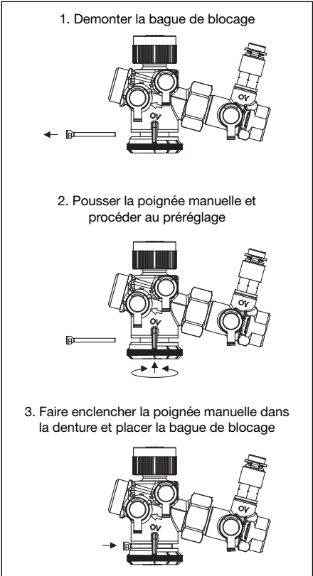
Fig. 7.1 Réglage du débit
