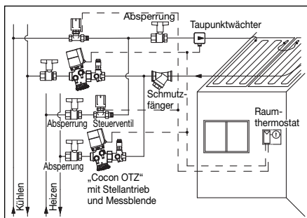
Abb. 6.2 Vierleitersystem
