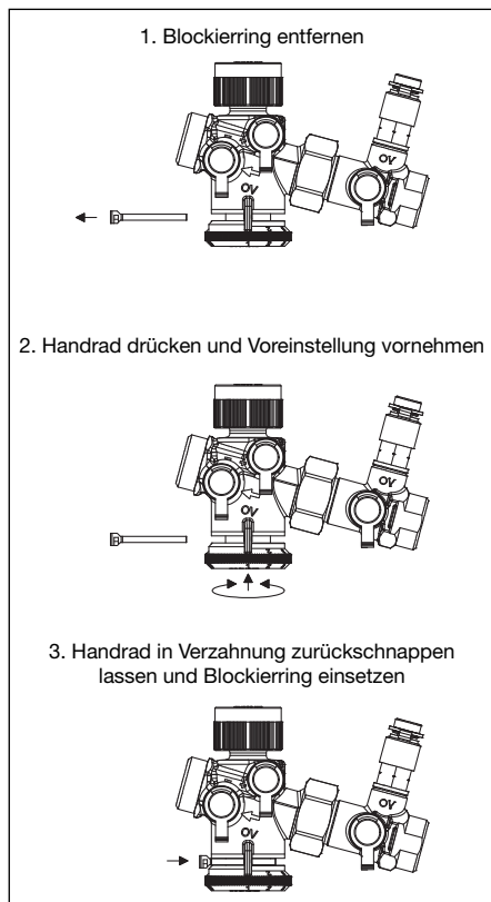
Abb. 7.1 Durchflusseinstellung
