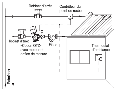
Fig. 6.1 Système à deux tuyaux
