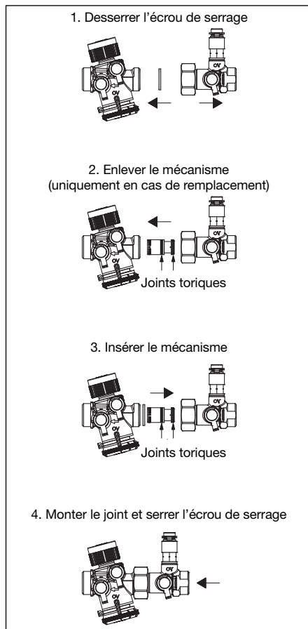
Fig. 6.3 Remplacement du mécanisme à l'orifice de mesure
