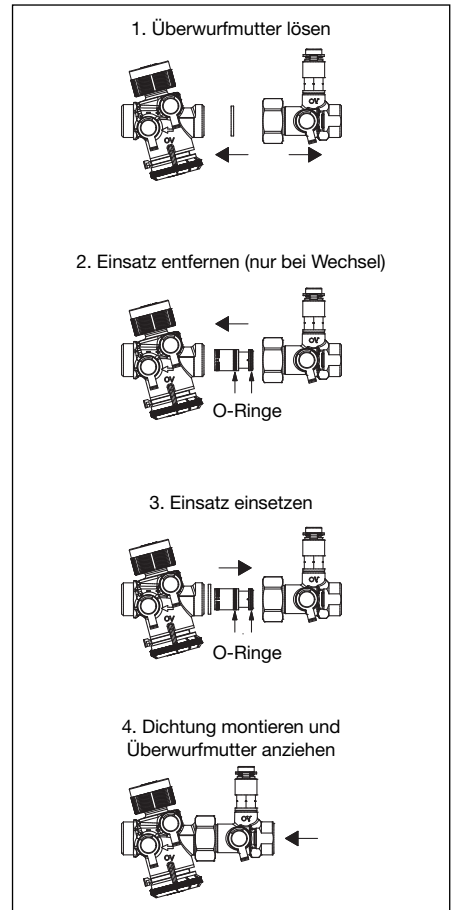
Abb. 6.3 Messblendeneinsatz wechseln
