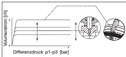
Abb. 5.6 Volumenstromkennlinie für unterschiedliche Voreinstellungen
