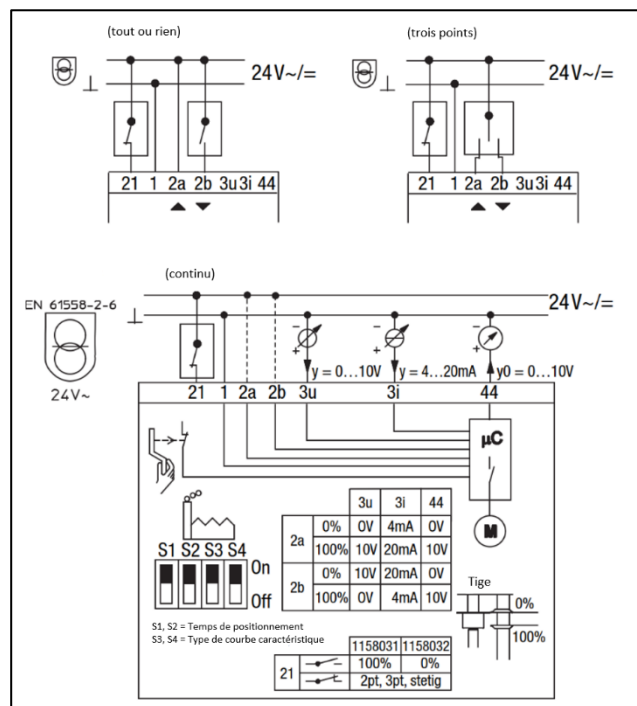
Schémas électriques réf. 1158031/32
