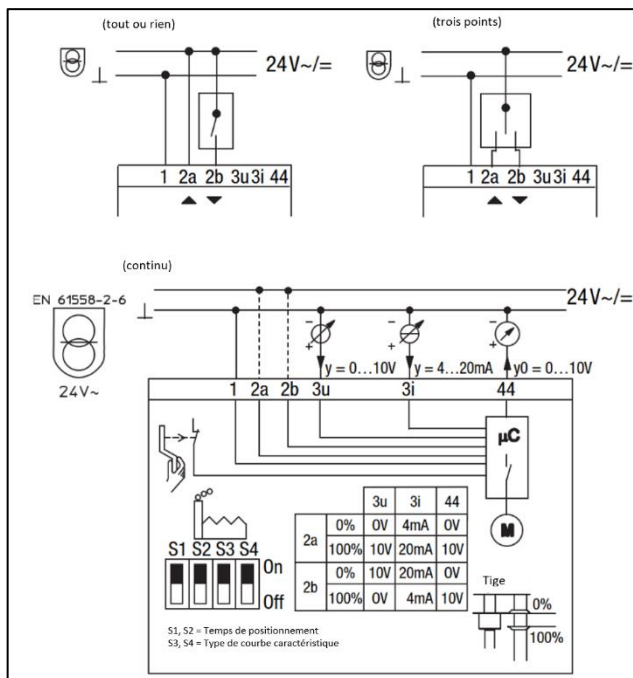
Schémas électriques réf. 1158030
