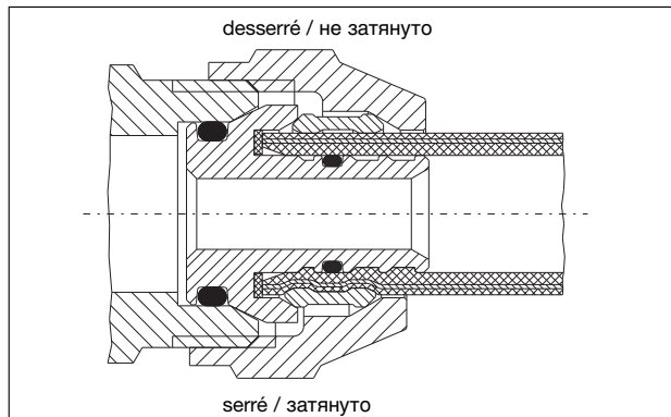
Ecrou et bague de serrage pour pièce à raccordement mâle Присоединение для наружной резьбы
