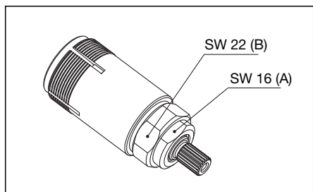
Abb. 6.3 Klemmoberteil
