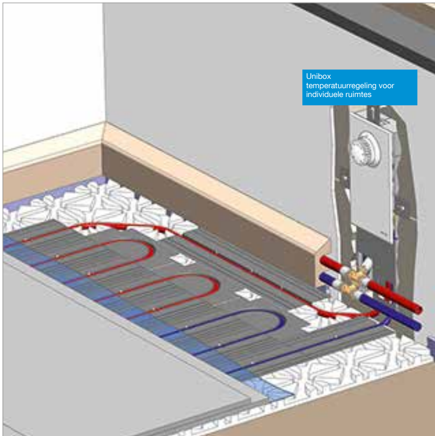
Unidis vloerverwarming in combinatie met plintverwarming en het Cofloor droogbouwstelsel
