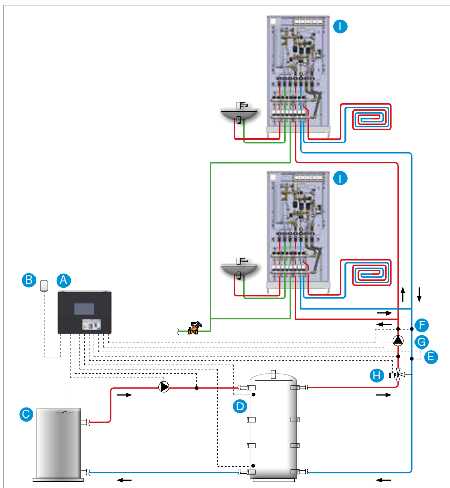
System opbouw
