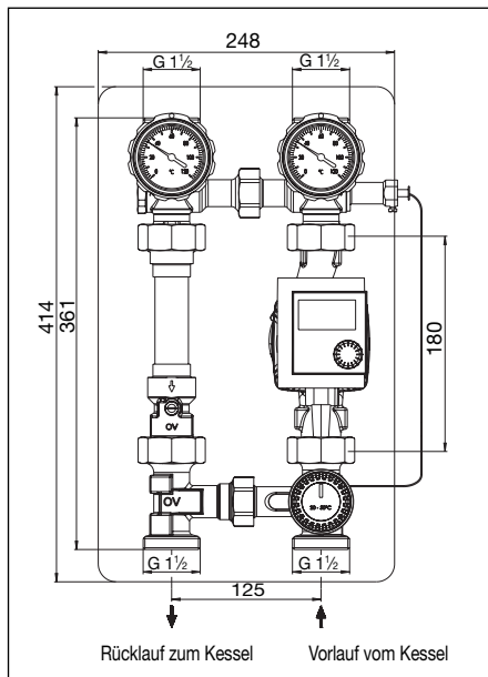
Abb. 4.3 Pumpengruppe „Regumat FR-180“
