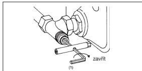
Obr. 3 Šroubení uzavřít
