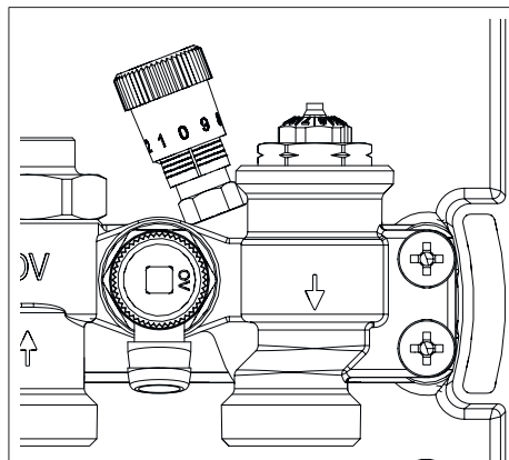
Fig. 4: Réglage du bypass
