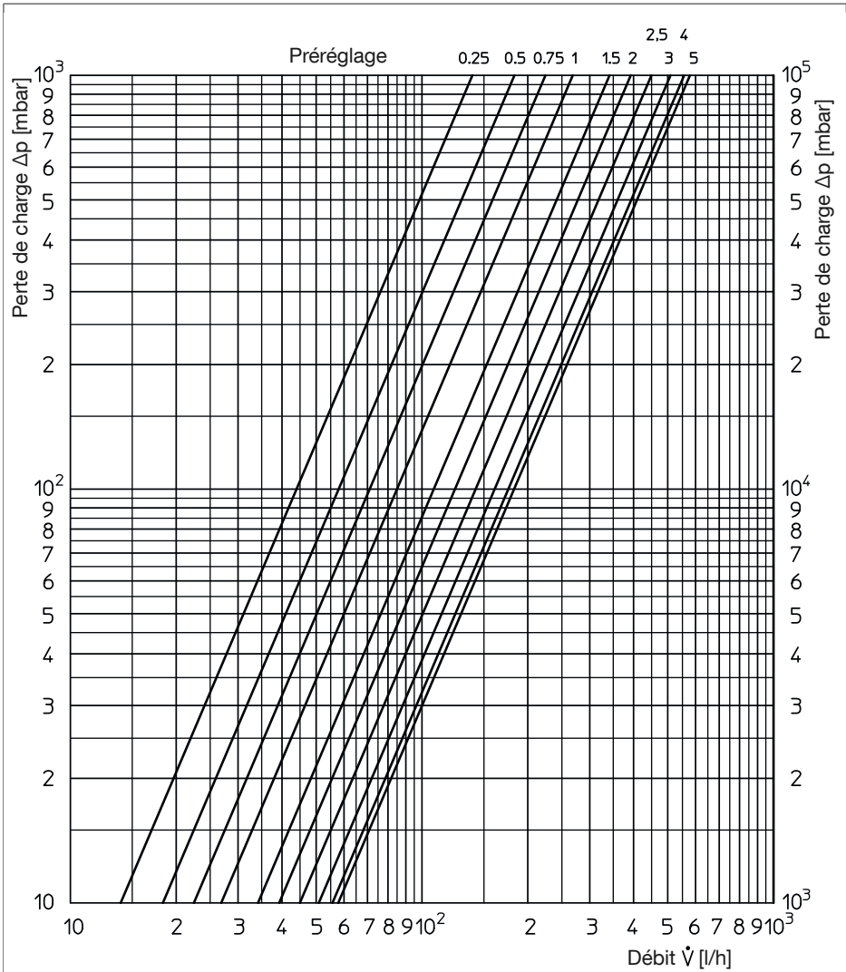
Fig. 13: Diagramme - Mécanisme de réglage avec un écart P de 2 K, bypass fermé
