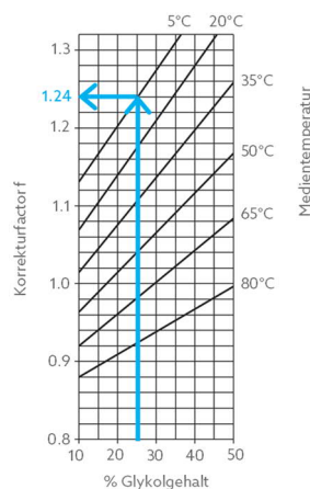
Korrekturfaktor f für Propylen Glykol
