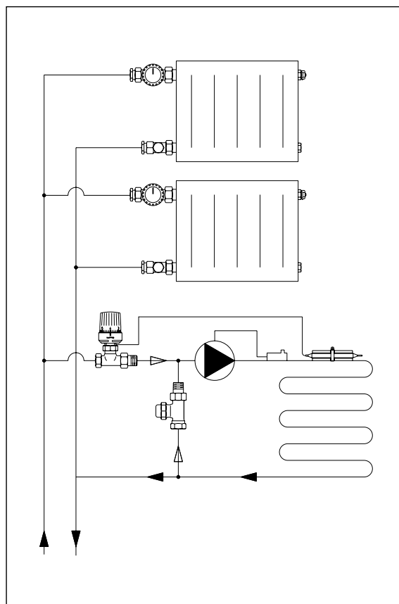
Montagevoorbeeld
