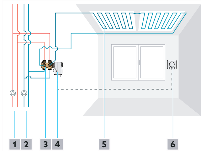
Fig. 1: Schéma d'installation
