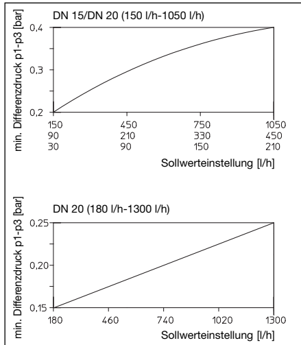
Abb. 5.7 Min. Differenzdruck / Sollwerteinstellung
