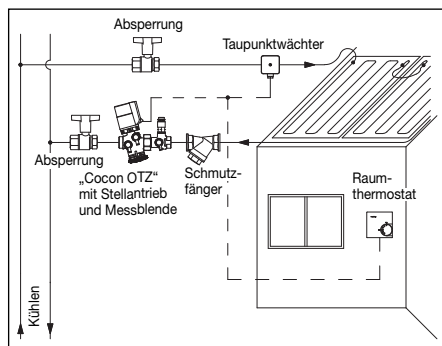
Abb. 6.1 Zweileitersystem
