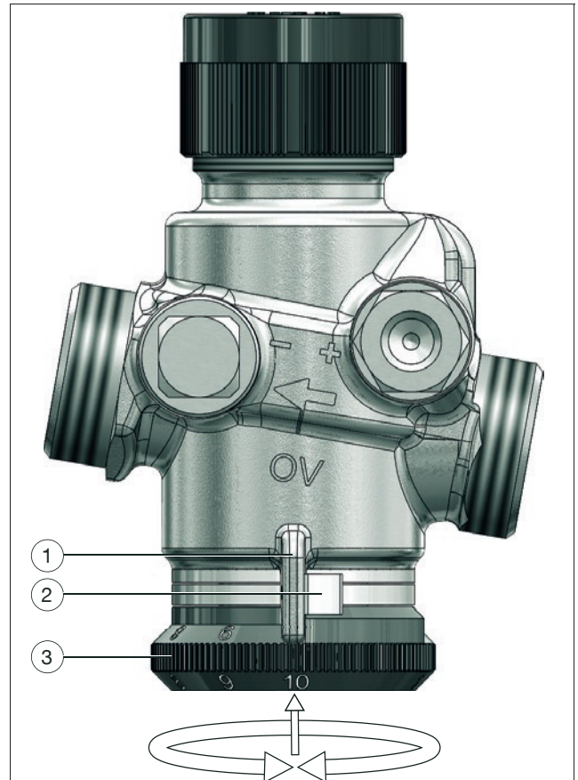
Abb. 6: Einstellen des Volumenstroms
