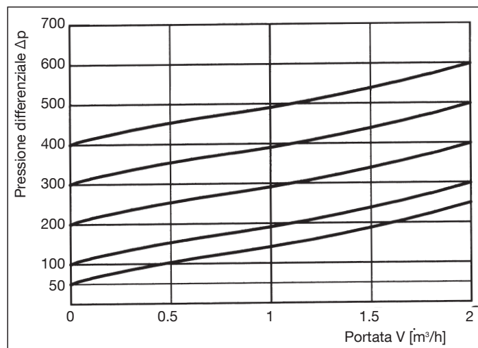
Diagramma delle portate con bypass (regolatore delle pressioni differenziali)
