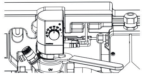
Abb. 2: Überwurfmutter befestigen
