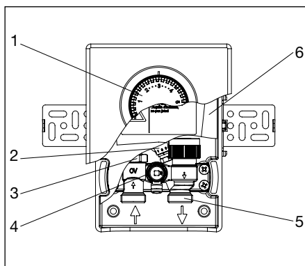
Abb. 4.1 Übersicht „Unibox E BV“
