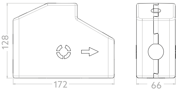
图 5： 绝缘壳
