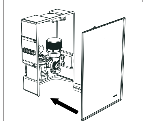
Fig. 10: Montage du capot
