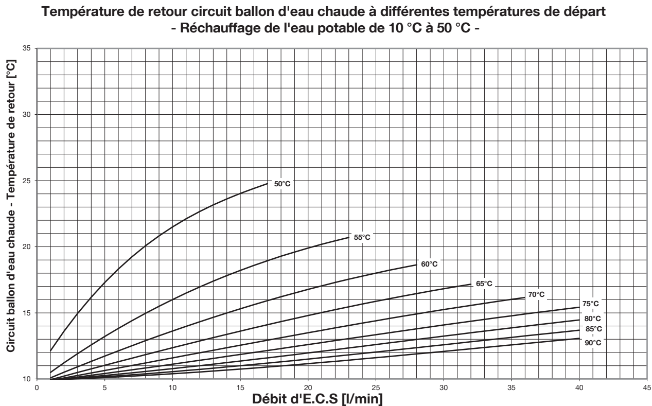
Fig. 45: Température de retour du circuit ballon d'eau chaude - Réchauffage de l'eau potable à 50 °C
