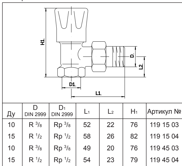
Угловой вентиль
