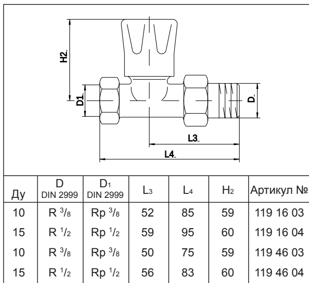
Прходной вентиль
