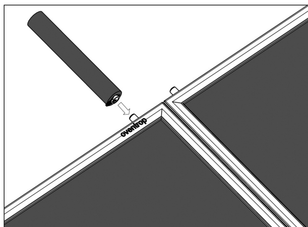
Abb. 4 Kollektorverbindungsleitung montieren: Kollektorverbindungsleitung auf den Kollektoranschluss schieben, Spannklemmer muss einrasten.
