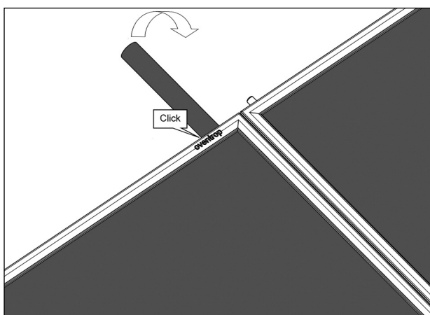
Abb. 5 Kollektorverbindungsleitung zum zweiten Anschluss biegen, auf den Anschluss schieben, Spannklemmer einrasten lassen.
