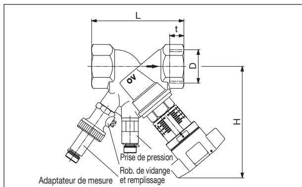
filetage femelle selon EN 10226 des deux côtés, réf. 10601..
