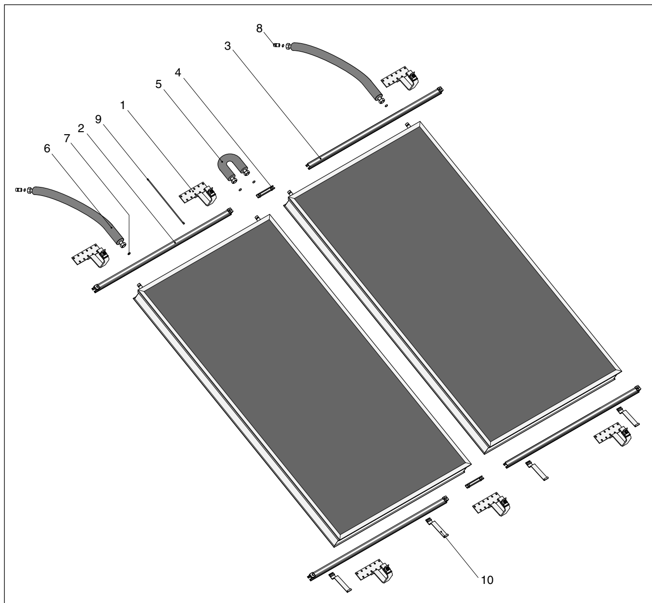
Grundset Aufdachmontage Art.-Nr. 136 12 80 (Kollektoren nicht im Lieferumfang enthalten)
