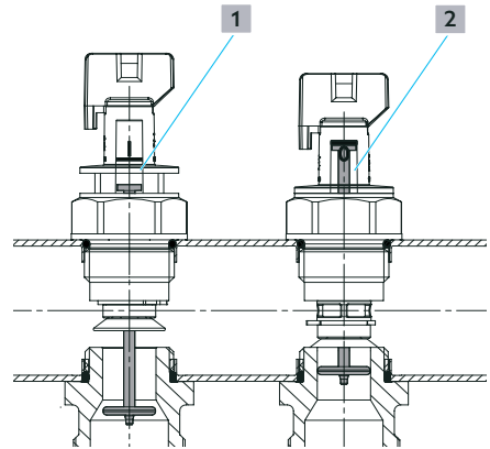
Fig. 5: Einstellung Durchflussindikator
