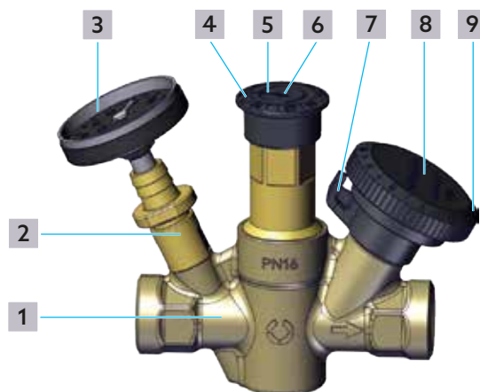
Afb. 1: Opbouw
