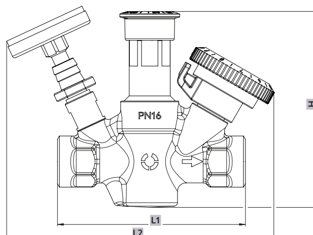
Afb. 2: Afmetingen lateraal
