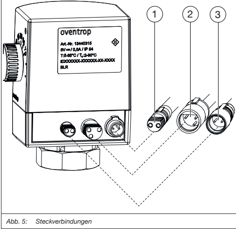
Abb. 5: Steckverbindungen
