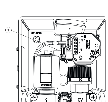
Abb. 10: Funkempfänger „R-CON FBH“ elektrisch anschließen
