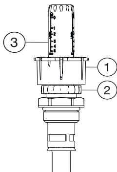
Fig. 3: Construction mécanisme de mesure et de réglage du débit
