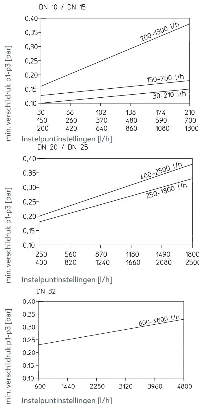
Afb. 13: Minimale verschillendrukken
