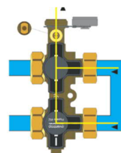
Fermeture et vidange du côté appareil
