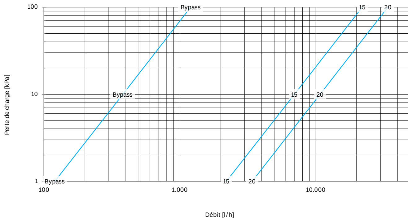
Diagramme de perte de charge
