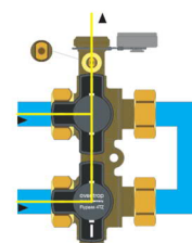
Remplissage et purge du côté installation
