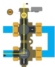
Vidange et purge du côté installation et du côté appareil, rinçage du côté installation
