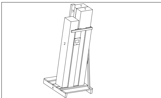
Abb. 1: Verpackungseinheit OKP 20
