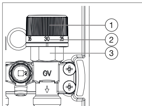
Abb. 4: Handrad
