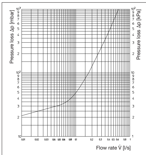
Diagramma delle portate „Regumat F-130/F-180/FR-180”
