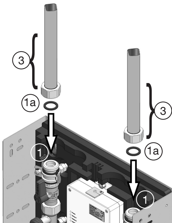
Abb. 31: Montage „Regudrain Duo“ in Reihenleitung
