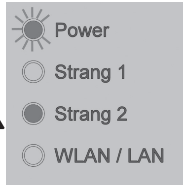
Abb. 110: Blink-Code für Störung im Spülbetrieb (S2)
