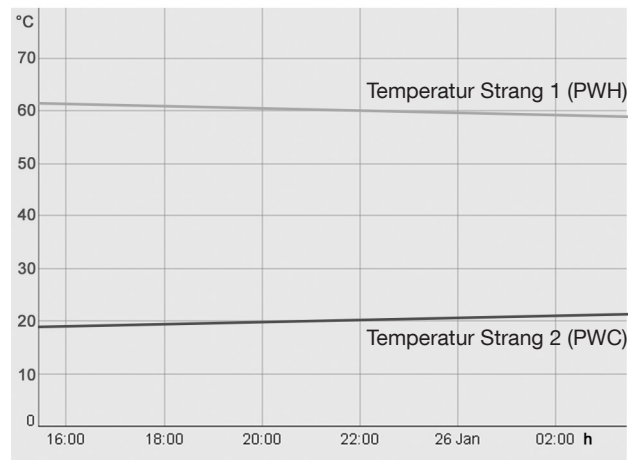
Abb. 108: Beispiel für erfasste Temperaturwerte auf Tagesbasis
