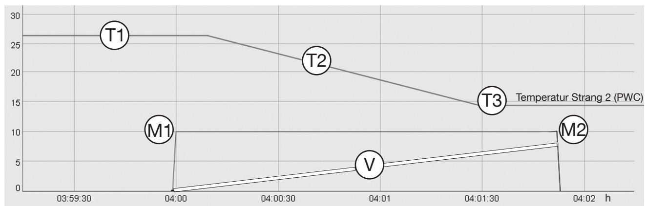
Abb. 109: Temperaturveränderung nach eingeleiteter Spülung (Detailansicht)
