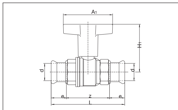
Dimensions item no. 1077162 – 66 (Ø 15 – Ø 35),
