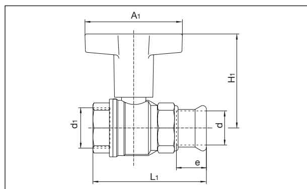
Dimensions item no. 1077152 – 56 (G 1/2 x Ø 15 – G 1 1/4 x Ø 35),
