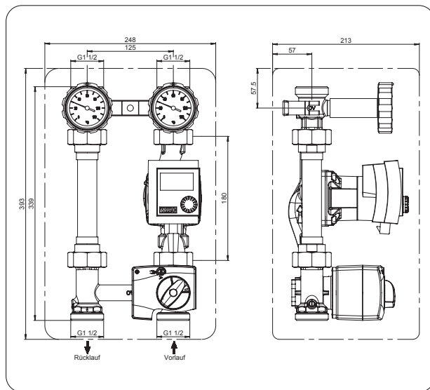
„Regumat M3-180“ DN 25 – kurze Bauform
