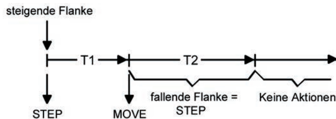
Bild 16: Bedienkonzept "Kurz-Lang-Kurz"
