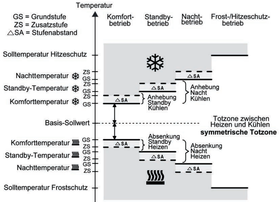
Bild 39: Solltemperaturen in der Betriebsart "Grund- und Zusatzheizen und -kühlen" mit symmetrischer Totzone
